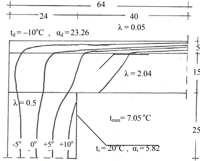
Şekil 4. Teras kat örneği (Yücesoy, 1990)
