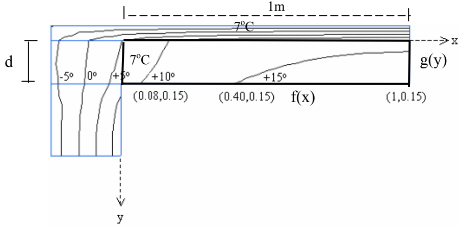
Şekil 5. Teras kat örneği için (Şekil 4'deki) QuickField programından elde edilen izoterm eğrileri ve incelenen sistemin sınır-değer probleminin çözümünde kullanılacak basitleştirilmiş gösterimi
