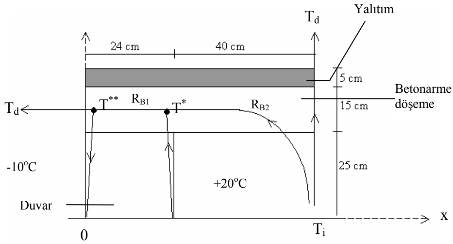
Şekil 6. İncelenen kesit için ısı akışı yolları
