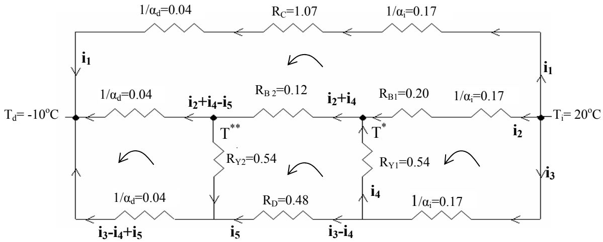
Şekil 7. Şekil 6’deki kesit için tanımlanan elektrik devresi
