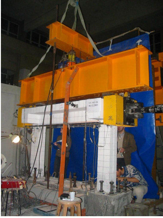
Şekil 3. Deney düzeneği
